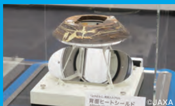
背面ヒートシールド(実物)
